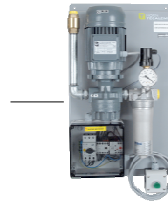
电动吸油泵
